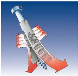
Βύσματα διαφόρων τύπων
