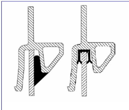
ΚΟΛΛΗΤΗ ΕΝΩΣΗ ή ΕΛΑΣΤΙΚΟ ΠΑΡΕΜΒΥΣΜΑ
