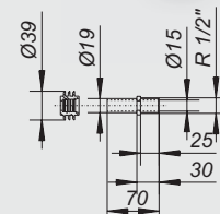
Urinal-Zulaufset iQ Universal
