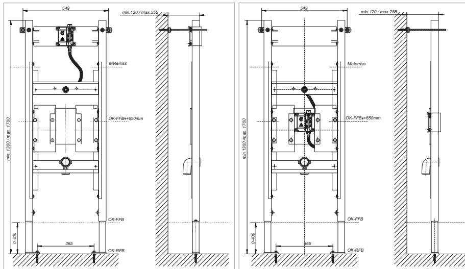
Rohbauset iQ R 1
