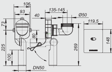
Elektronikset iQ 145 ET 1 für „Taro“/„Tamaro“
