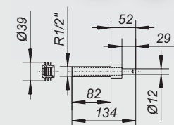
Urinal-Zulaufset iQ Taro/Tamaro
