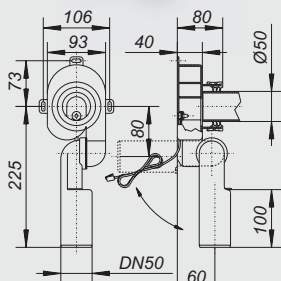
Urinal-Absaug-Siphon HL 430 E
