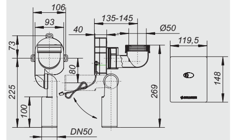
Elektronikset iQ 110 ET 1 für „Taro“/„Tamaro“
