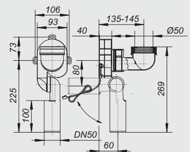
Elektronikset iQ 110 ET 2 für „Taro“/„Tamaro“
