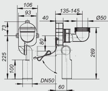
Elektronikset iQ 145 ET 2 für „Taro“/„Tamaro“
