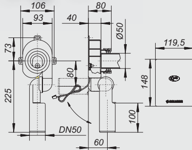
Elektronikset iQ 145 E 1
