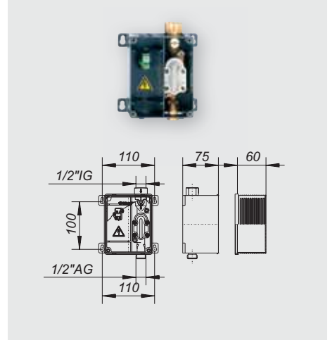
Rohbauset iQ R 2
