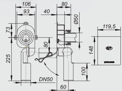
Elektronikset iQ 110 E 1
