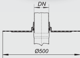
Rohrdurchführung DallBit
