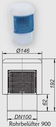
Rohrbelüfter 900
