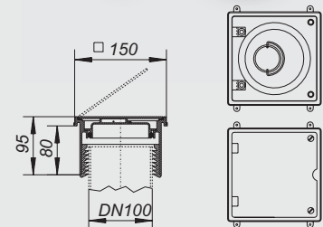
Reinigungsverschluss (SML-Anschluss)
