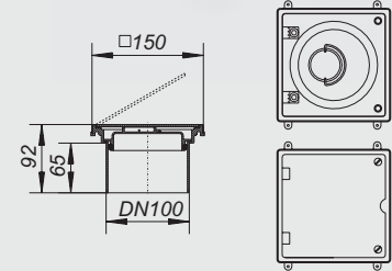
Reinigungsverschluss
